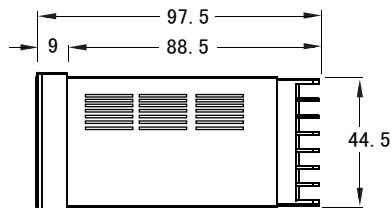
侧面尺寸 Side face size
